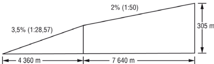
Bild 13. Start/stigyta för instrument-FATO.
