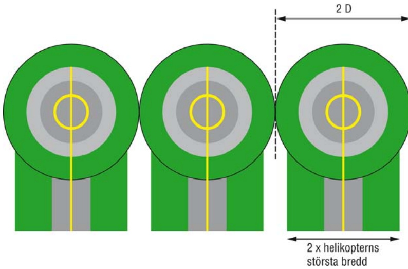
Bild 7. Uppställningsplatser för helikopter som ska användas vid sväng under hovring och samtida rörelser.
