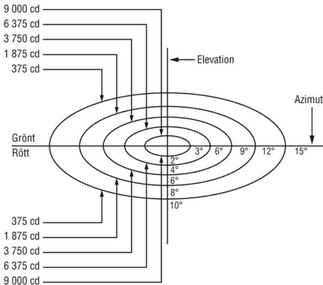
Bild 28d. Isocandeladiagram för ljus på helikopterflygplats.
