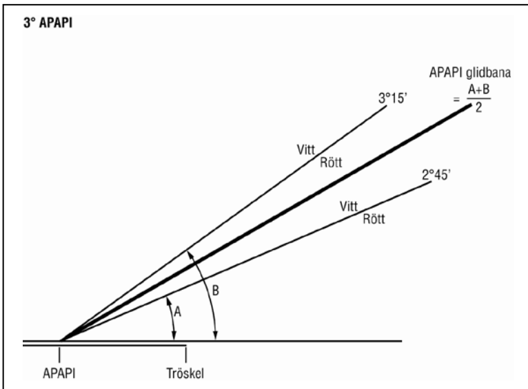
Bild 35. Glidbanevinklar APAPI
