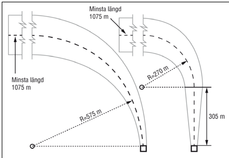
Bild 10. Inflygnings- och start/stigytor avsedda för sväng in- och utflygning för samtliga FATO och FATO/TLOF.
