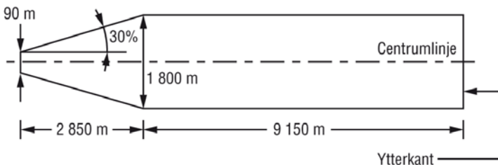
Bild 12. Övergångsyta för FATO eller FATO/TLOF där PinS-metoden med visuellt segment används samt övergångsyta för instrument-FATO eller FATO/TLOF avsett för precision och icke-precisionsflygning.
