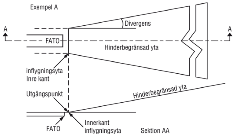
Bild 33. Hinderbegränsande yta för visuellt glidbanestöd.
