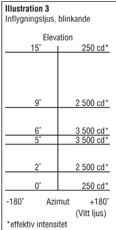
Bild 28c. Isocandeladiagram för ljus på helikopterflygplats.
